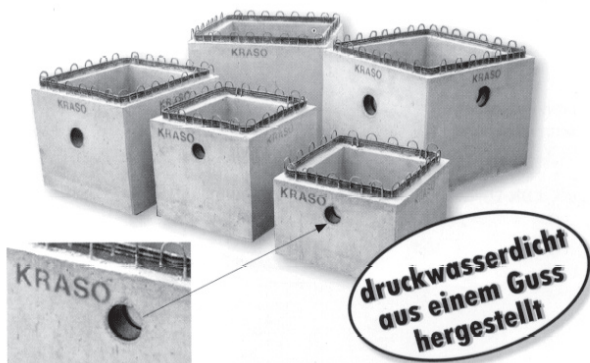
Druckwasserdichter KRASO® Rohranschluss*
