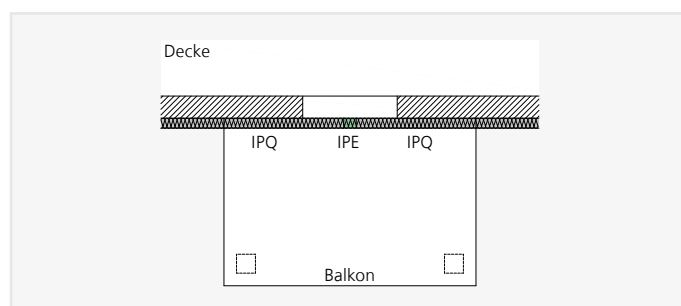
ISOPRO® IPE – Gestützter Balkon mit hohen Horizontalkräften
