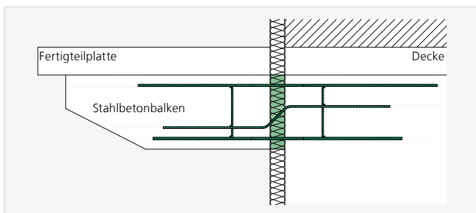
ISOPRO® IPTS – Einbauschnitt mit Fertigteilplatten
