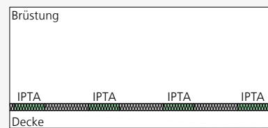
ISOPRO® IPTA – Ansicht aufgesetzte Brüstung
