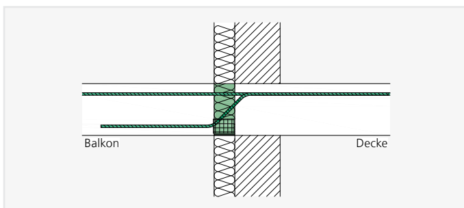
ISOPRO® IP EL/ER – Einbauschchnitt cv35
