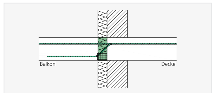
ISOPRO® IP EL/ER – Einbauschchnitt cv50
