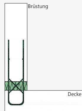
ISOPRO® IPTA – Einbauschnitt aufgesetzte Brüstung
