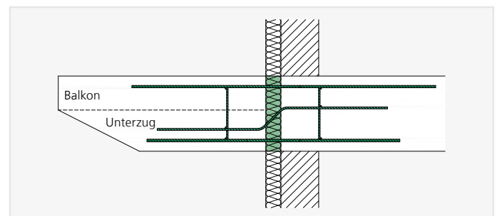
ISOPRO® IPTS – Einbauschnitt mit monolithisch mit der Balkonplatte verbundenen Unterzügen
