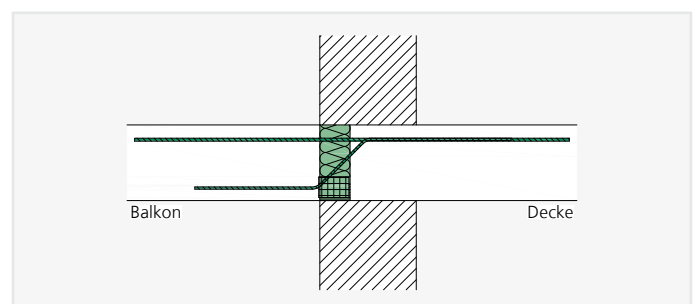
ISOPRO® IP – Einbauschchnitt einschaliges Mauerwerk
