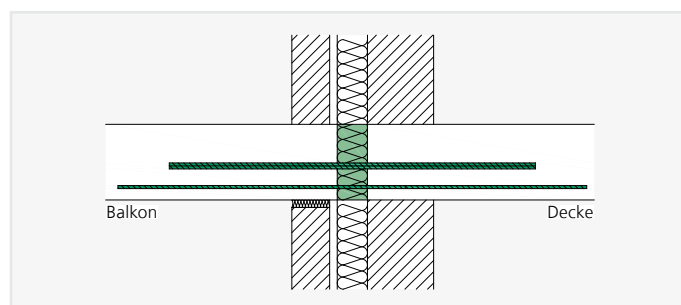
ISOPRO® IPE – Einbauschnitt zweischaliges Mauerwerk
