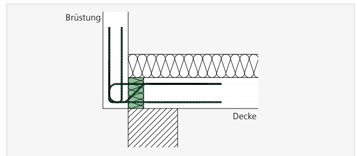
ISOPRO® IPTF – Einbausschnitt einer vorgesetzten Brüstung mit einschaligem Mauerwerk
