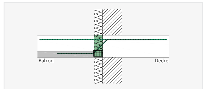
ISOPRO® IP 2-teilig – Einbauschchnitt Wärmedämmverbundsystem
