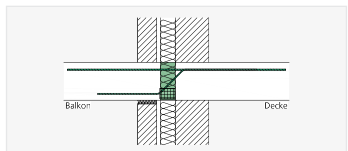
ISOPRO® IP – Einbauschchnitt zweischaliges Mauerwerk
