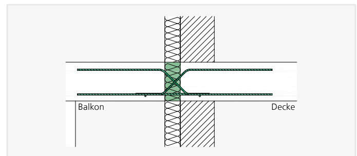
ISOPRO® IPTQQ, IPTQQS – Einbauschchnitt Wärmedämmverbundsystem – Querkraftstab deckenseitig gerade
