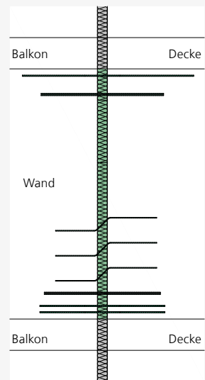
ISOPRO® IPTW – Einbauschchnitt mit monolithisch mit der Balkonplatte verbundener Wandscheibe
