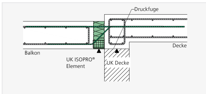
ISOPRO® Elemente bei Ort betonbauweise und höhenversetzten Deckenplatten
