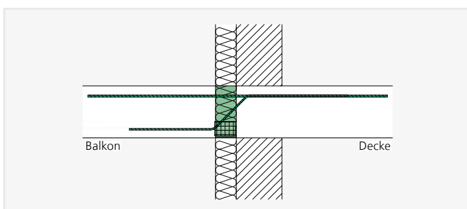
ISOPRO® IP – Einbauschchnitt Wärmedämmverbundsystem
