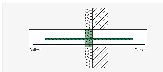
ISOPRO® IPE – Einbauschnitt Wärmedämmverbundsystem
