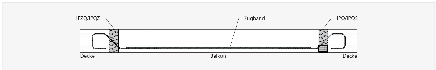
ISOPRO® IPZQ/IPQ, IPQZ/IPQS – Baueitiges Zugband in der unteren Bewehrungslage – Querkraftstab Ø 6 deckenseitig geschlauft
