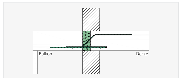
ISOPRO® IPTQS – Einbauschchnitt einschaliges Mauerwerk
