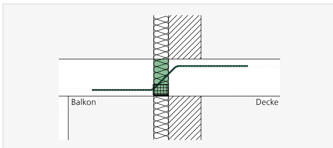
ISOPRO® IPQ, IPQS – Einbauschchnitt Wärmedämmverbundsystem
