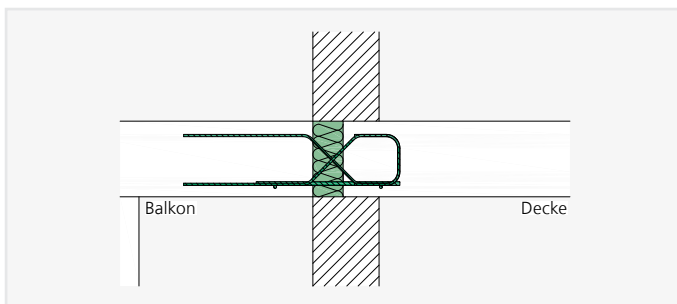
ISOPRO® IPTQQ – Einbauschchnitt einschaliges Mauerwerk – Querkraftstab deckenseitig geschlauft
