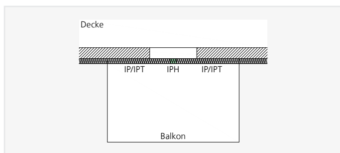
ISOPRO® IPH – Ausragender Balkon mit planmäßig auftretenden Horizontallasten
