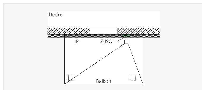
ISOPRO® Z-ISO – Balkon auf Stützen – Z-ISO Elemente im Bereich der Aussparung für die Entwässerung
