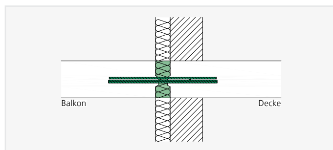
ISOPRO® IPH 3 – Einbauschchnitt im Wärmedämmverbundsystem
