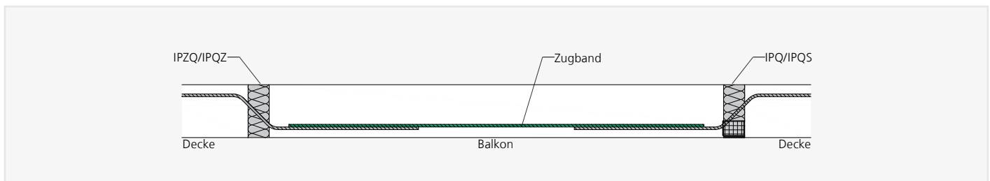
ISOPRO® IPZQ/IPQ, IPQZ/IPQS – Baueitiges Zugband in der unteren Bewehrungslage – Querkraftstab deckenseitig gerade
