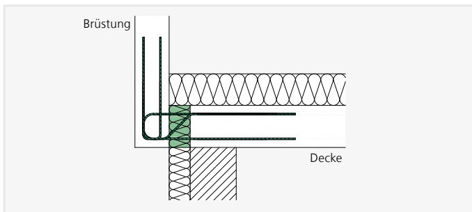
ISOPRO® IPTF – Einbausschnitt einer vorgesetzten Brüstung mit Wärmedämmverbundsystem
