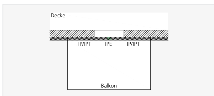
ISOPRO® IPE – Auskragender Balkon mit abhebenden Momenten
