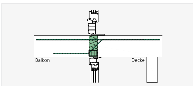
ISOPRO® IP – Einbauschchnitt Glasfassaden
