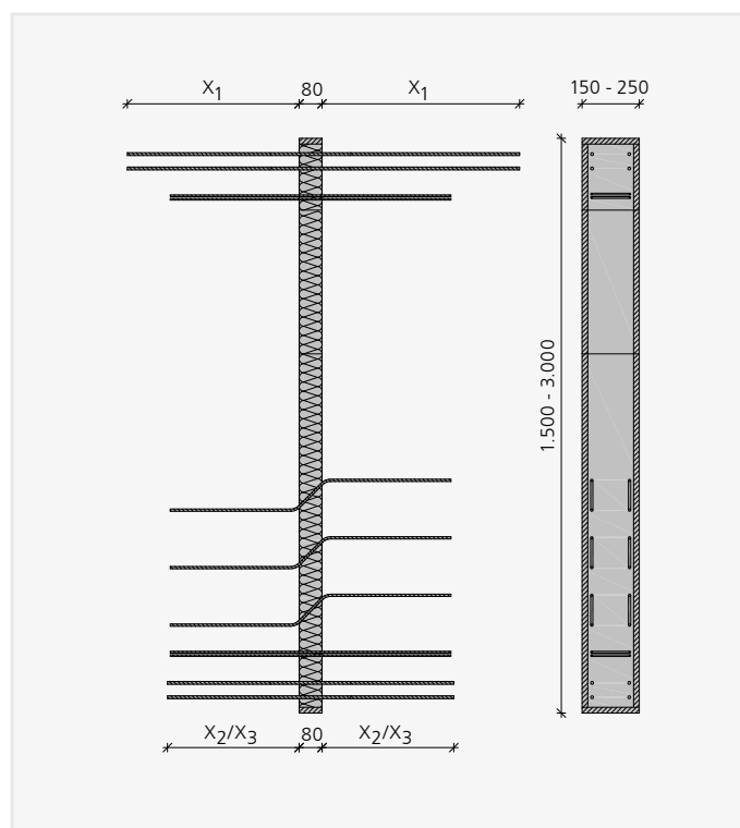
ISOPRO® IPTW – Ausführung mit Brandschutzplatten – R 90
