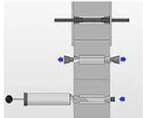
System mit Quellvergussmörtel
